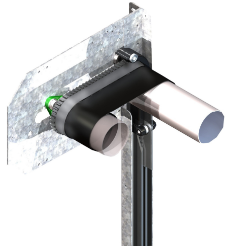
Direktdrift av portduken, Push and Pull teknologi.
