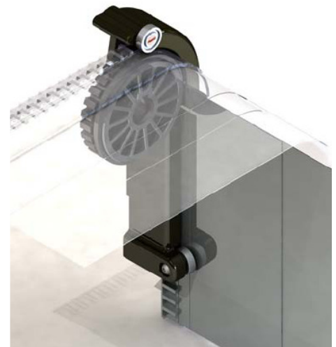
Återföringsbeslaget, för automatisk lagning av påkörd duk.
